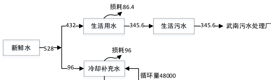
图 2-1 验收项目水平衡图 (t/a)
