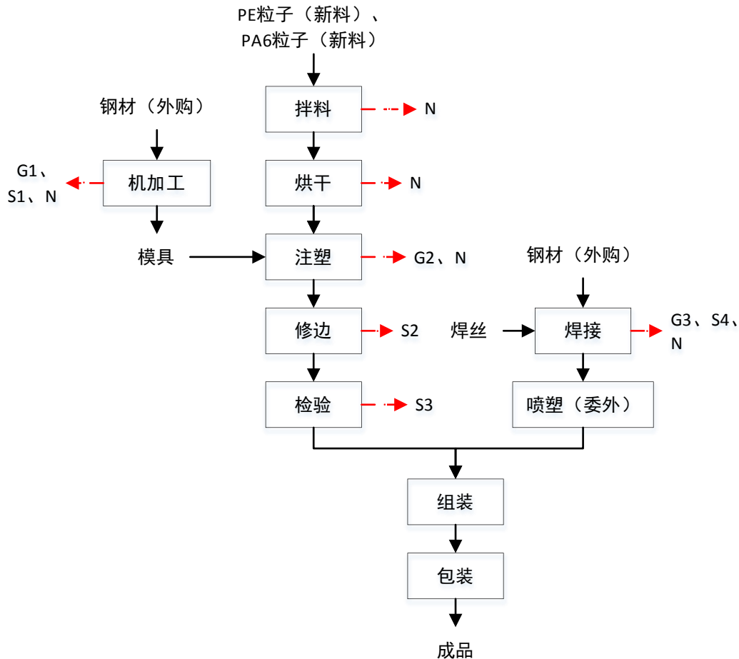
图 2-2 家具配件工艺流程图
