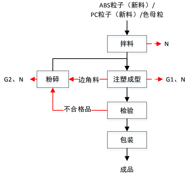
图 2-2 医疗器械零部件工艺流程图
