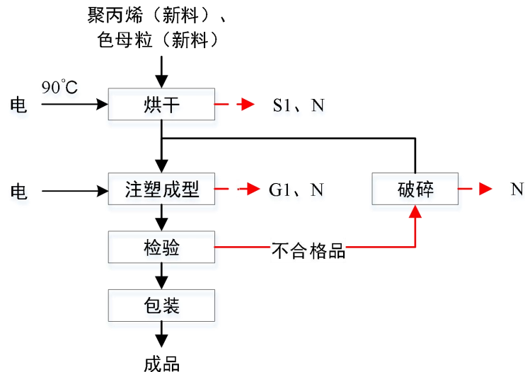
图 2-3 汽车电机骨架、电动车电机骨架生产工艺流程图
