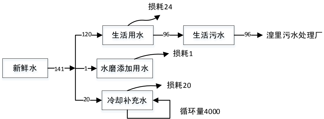
图 2-1 验收项目水平衡图 (t/a)
