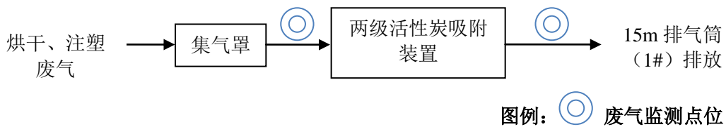
图 3-2 有组织废气处理流程图及监测点位
