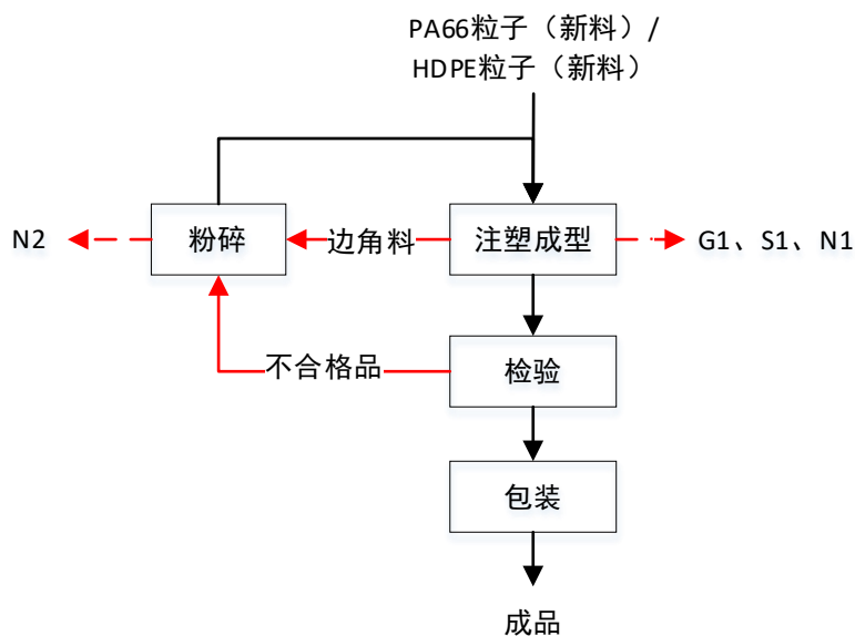
图 2-2 生产工艺流程图
