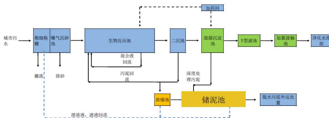
图 5-4 武南污水处理厂处理工艺流程
